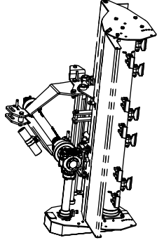
SISTEMA DE TRANSMISSÃO MONTADO
